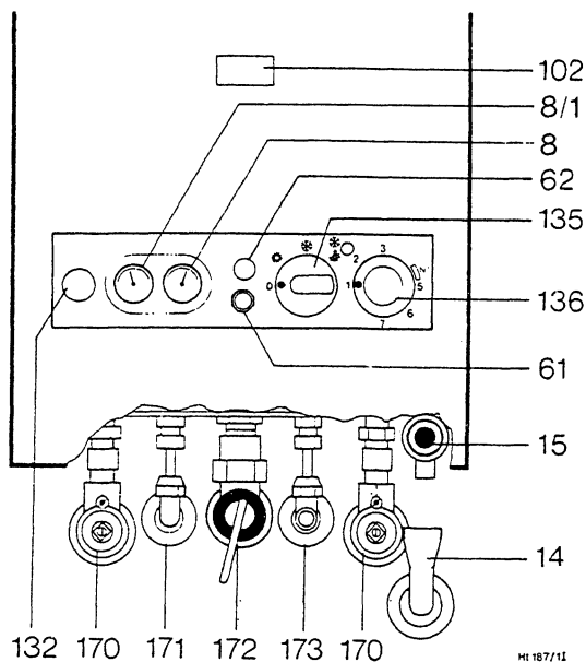
Fig. 10 Caldaia Combi
